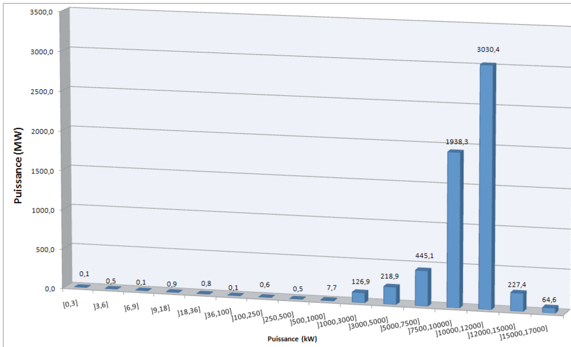
Répartition en puissance cumulée par tranche de puissance à fin décembre 2011 des installations de production éolienne raccordées au réseau ERDF
