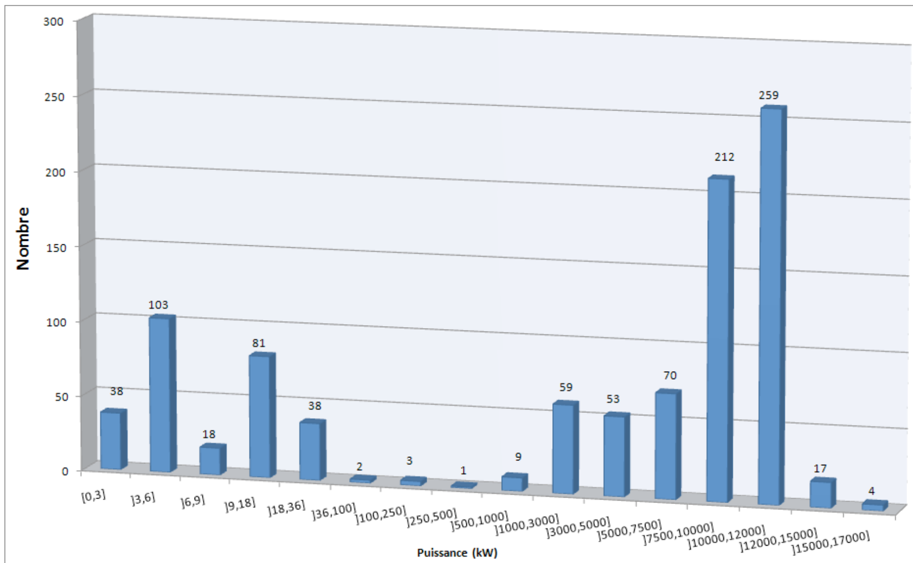
Répartition en nombre par tranche de puissance à fin décembre 2011 des installations de production éolienne raccordées au réseau ERDF
