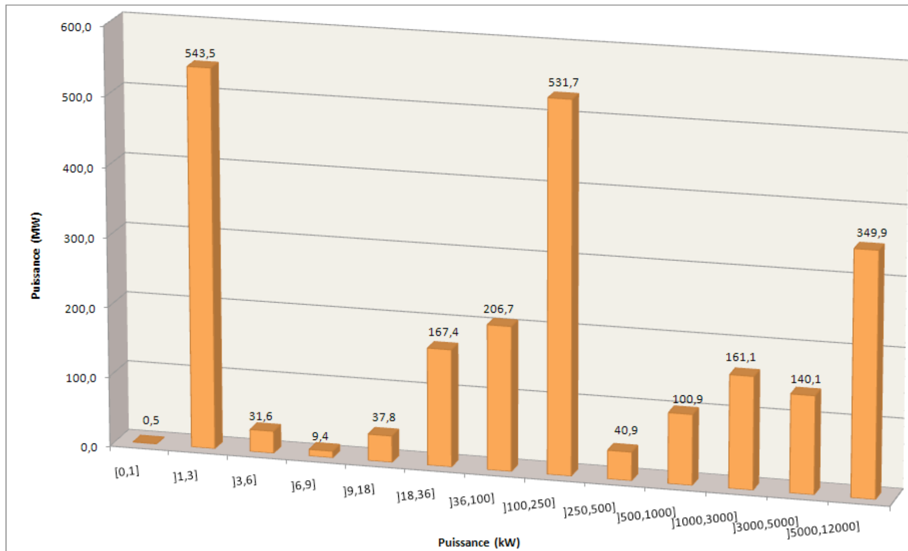
Répartition en puissance cumulée par tranche de puissance à fin décembre 2011 des installations de production photovoltaïque raccordées au réseau ERDF
